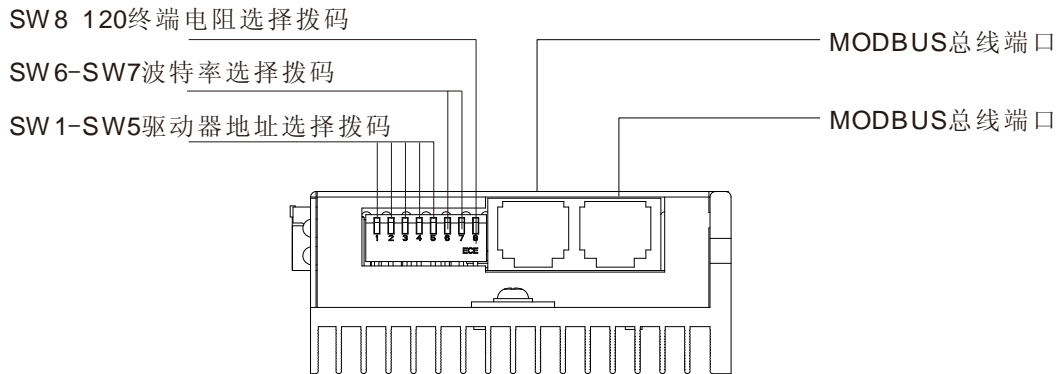
驱动器顶部接线示意图
