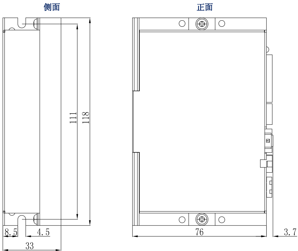
安装尺寸图（单位：mm）
