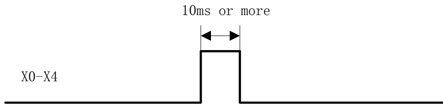
X0-X4 时序图
