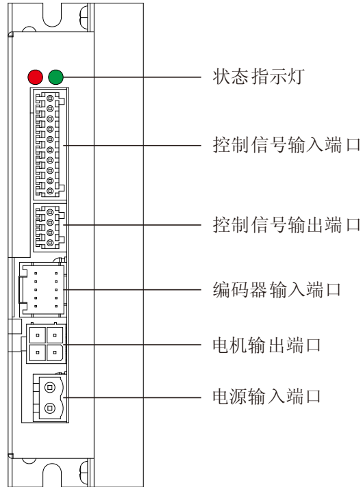
驱动器侧面接口示意图
